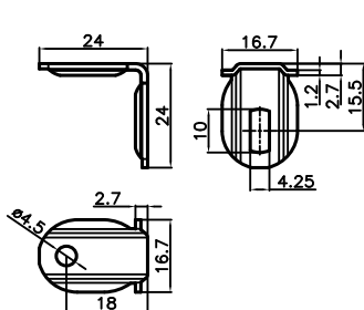
Złącze meblowe 1,2x24x24
