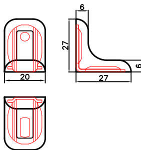
Złącze komplet
